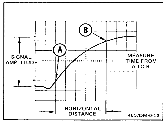
Fig. 19. Risetime.
