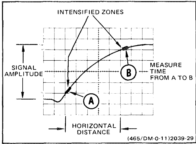
Fig. 28. Risetime.
