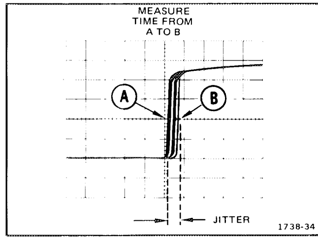
Fig. 23. Pulse jitter.
